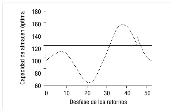
Figura 4 Dependencia de la capacidad de almacén óptima S respecto del desfase. Los puntos corresponden al sistema con retornos y la línea continua al sistema sin retornos
