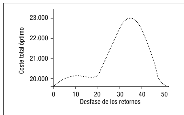
Figura 6 Dependencia del coste óptimo respecto del desfase
