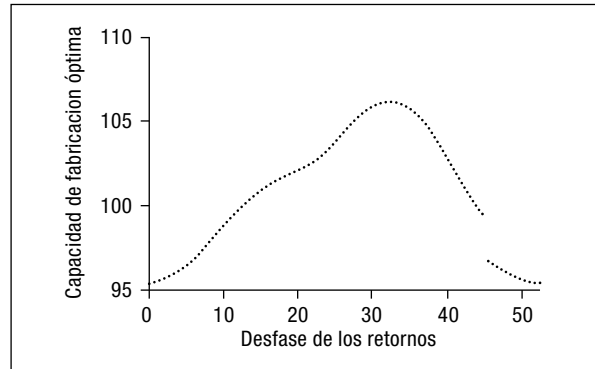
Figura 5 Dependencia de la capacidad de fabricación óptima respecto del desfase
